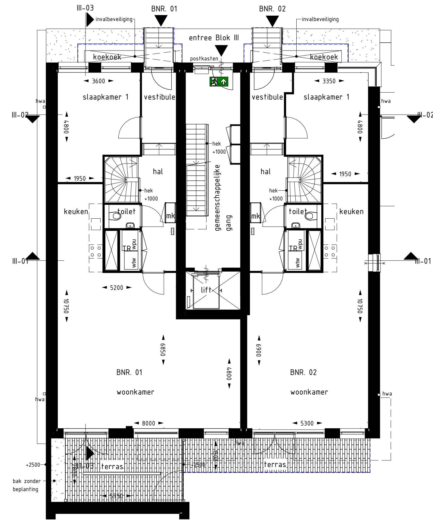
Begane grond Blok 3 1 : 100
