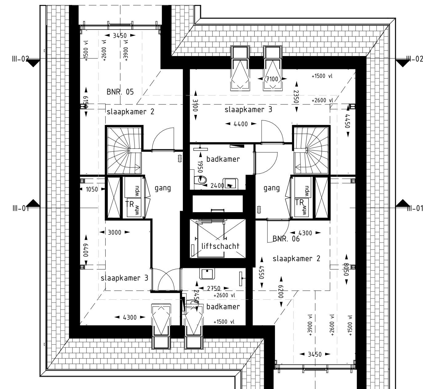
Derde verdieping Blok 3 1 : 100
