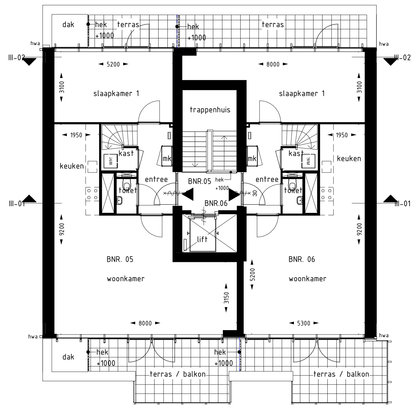
Tweede verdieping Blok 3 1 : 100
