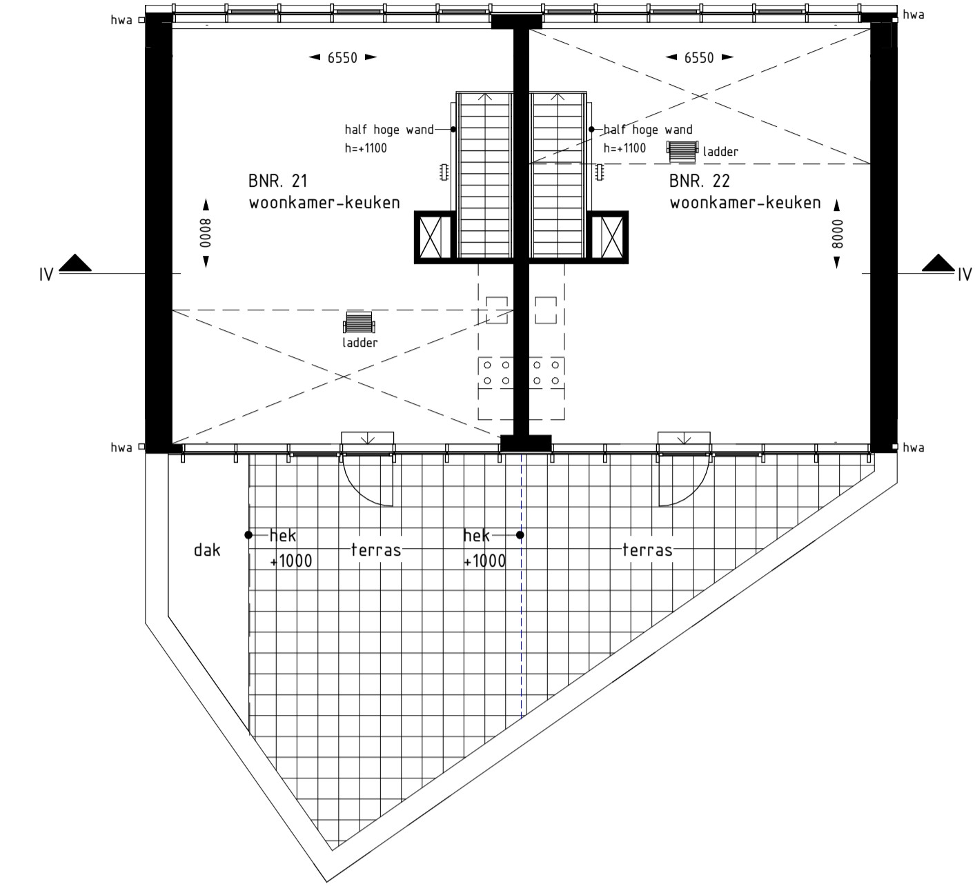
Tweede verdieping Blok 4 1 : 100
