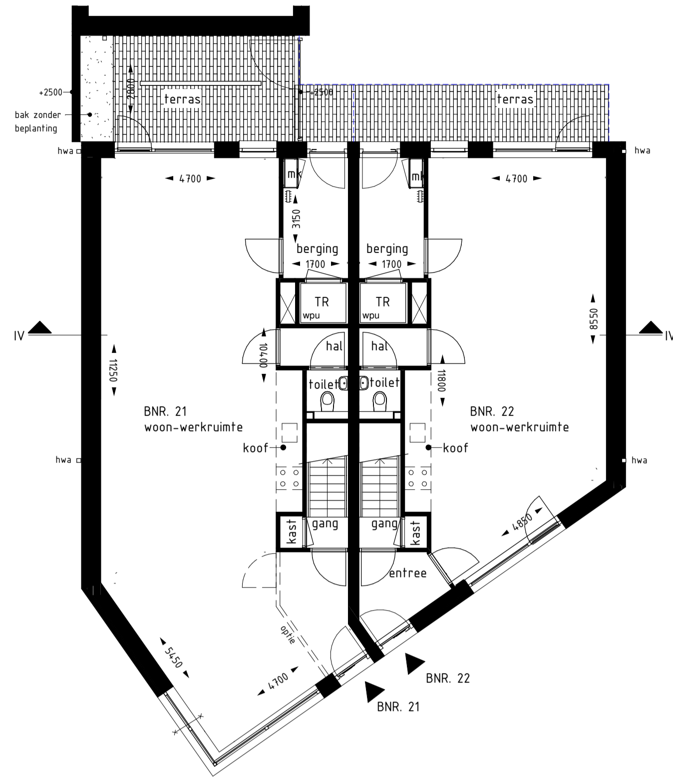
Begane grond Blok 4 1 : 100
