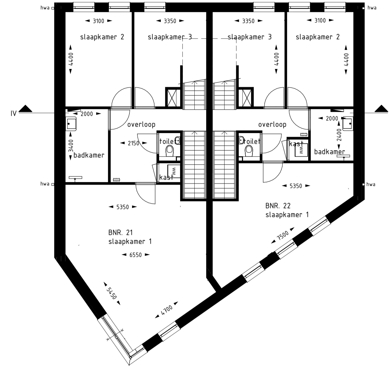
Eerste verdieping Blok 4 1 : 100
