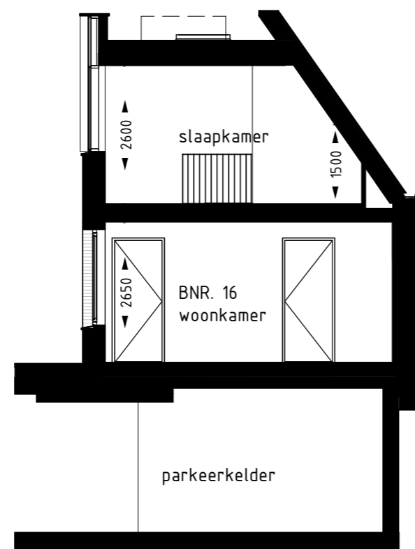
Doorsnede V-l Blok 5 west
