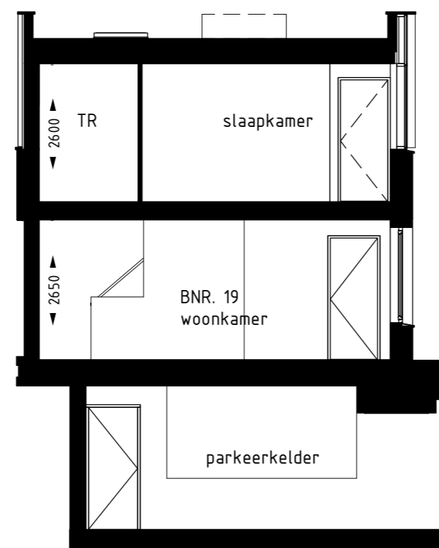
Doorsnede V-r Blok 5 oost
