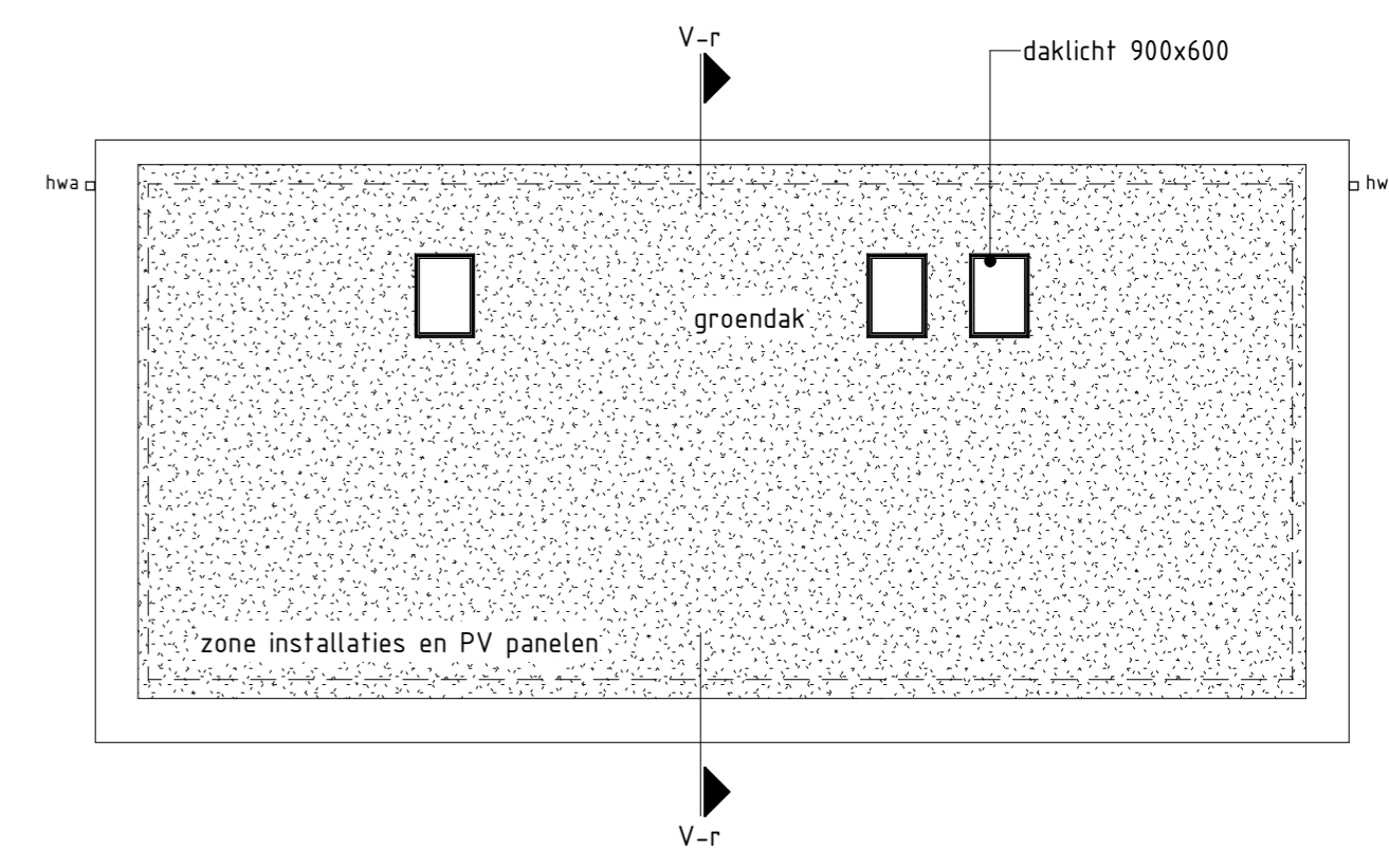
Dakoverzicht Blok 5 oost
