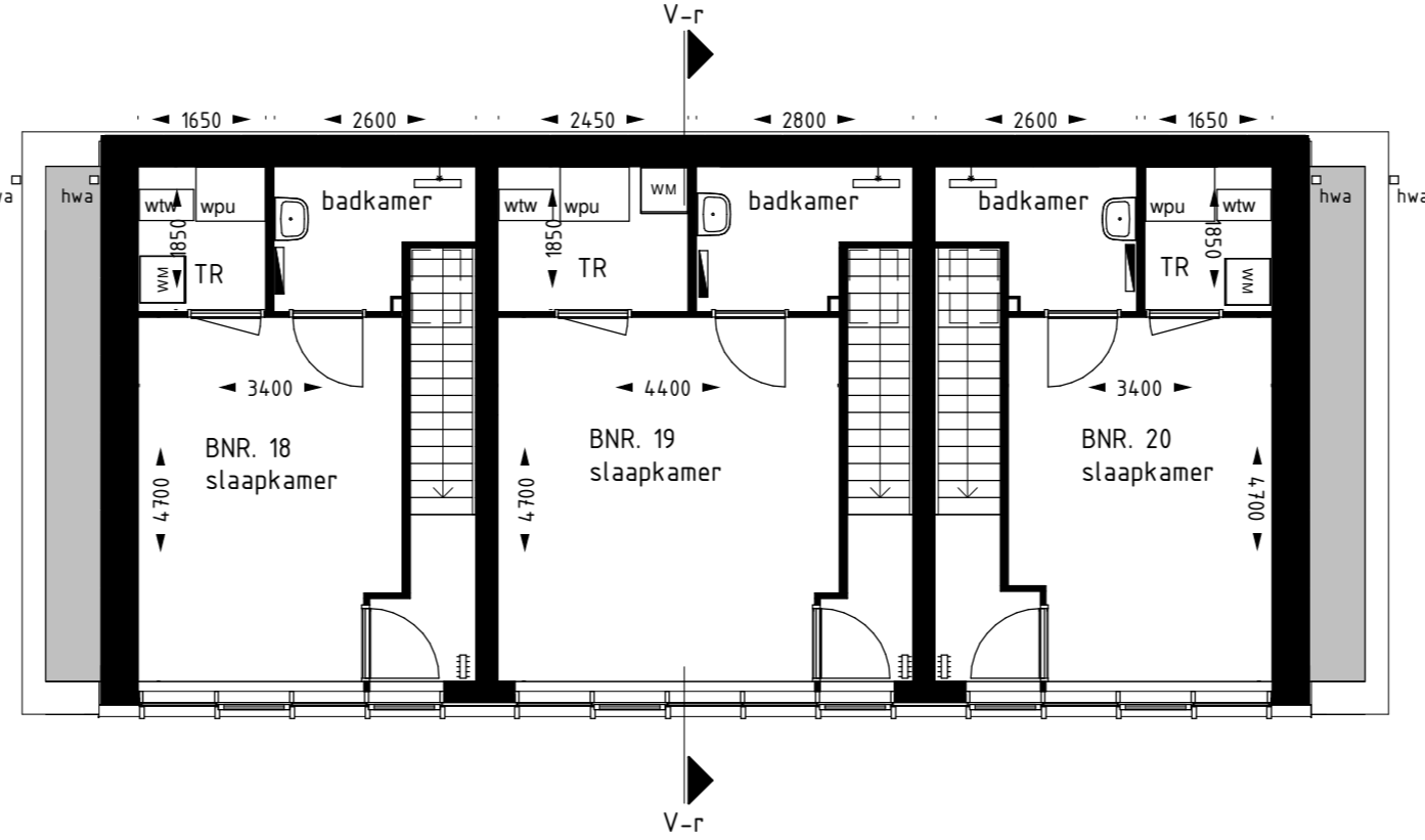
Eerste verdieping Blok 5 oost
