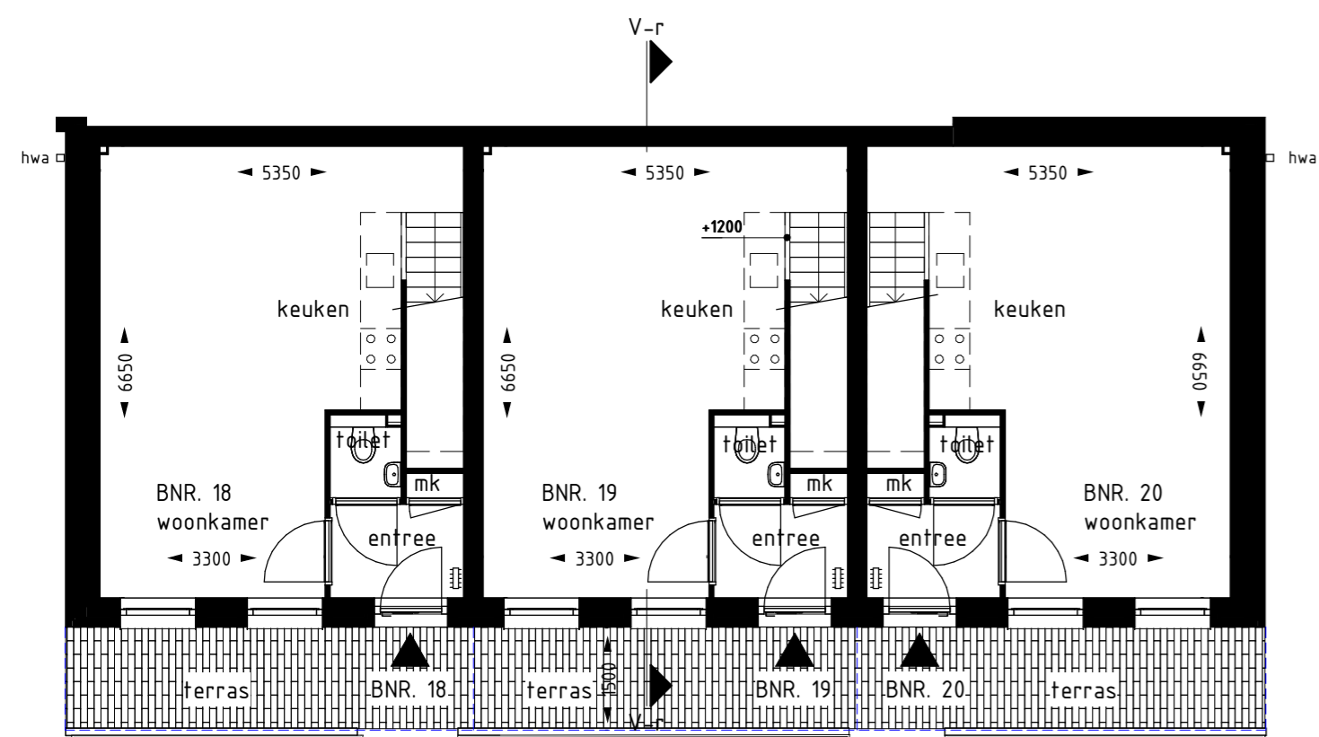
Begane grond Blok 5 oost
