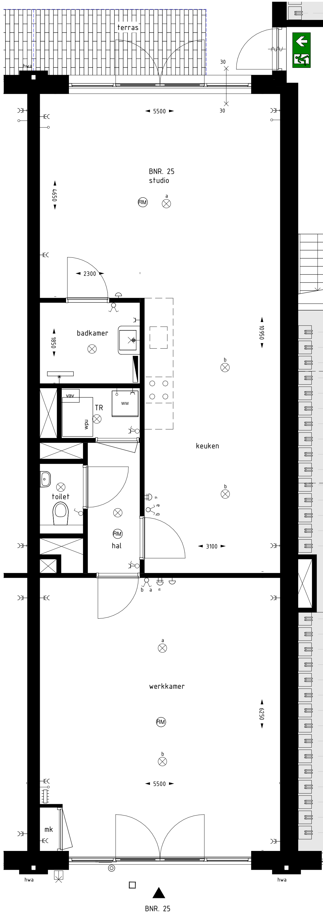
begane grond 1 : 50
